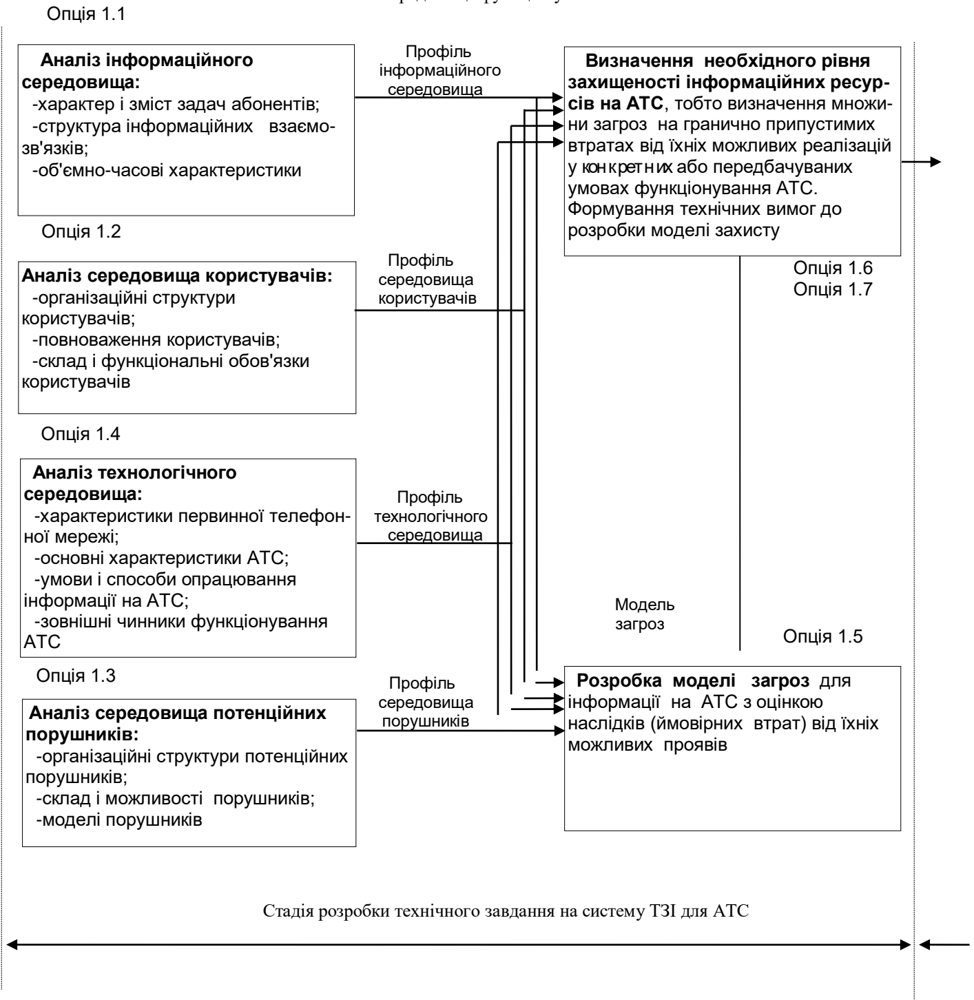
Рисунок 1- Схема організації робіт з ТЗІ на АТС
